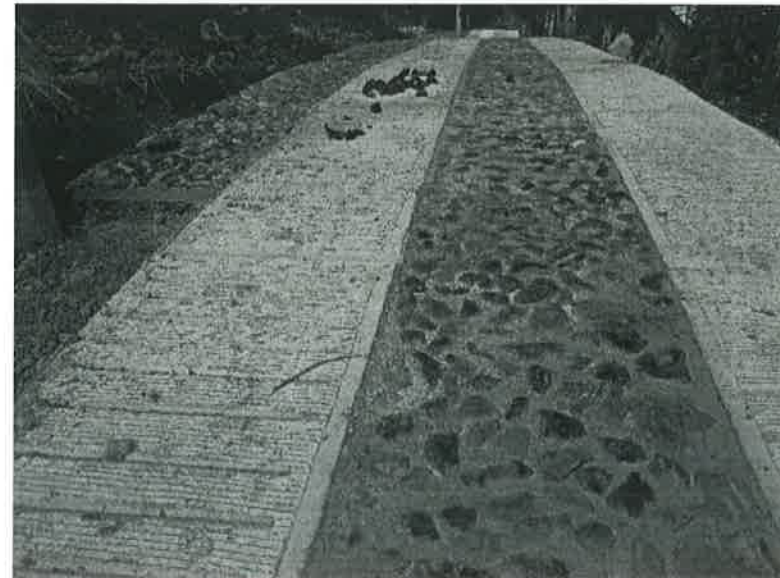
Concepto de obra ejecutado: Construcción de rampas de concreto hidraulico con huellas en acabado zampeado de 1.00m de ancho y 18 CM de espesor
