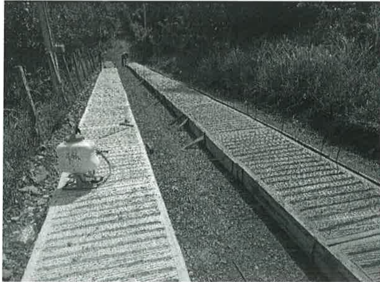
Concepto de obra ejecutado: Construcción de rampas de concreto hidraulico de 18 CM de espesor en rampad de 1.00m de ancho y fc=250kg/cm2
