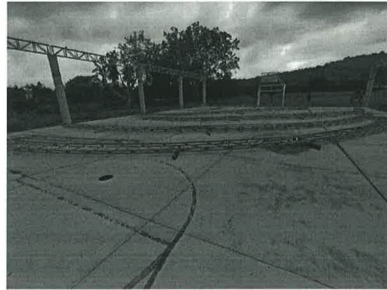
Consternados de cerchas a base de ángulo y perfil estructural.
