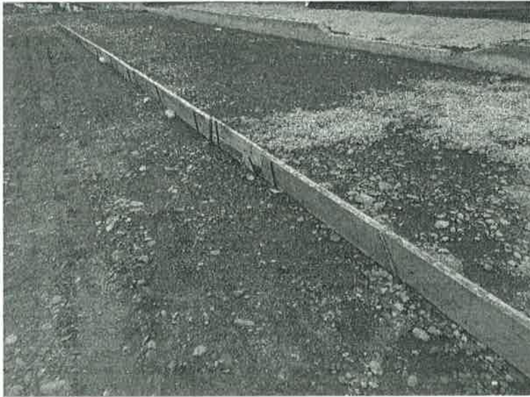
Colocación de cimbra en reglas y fronteras.
