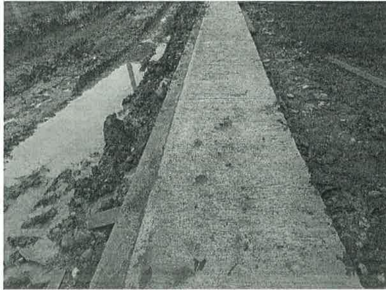
Concepto de obra ejecutado: Construcción de banqueta de concreto simple de 10 cm de espesor.
