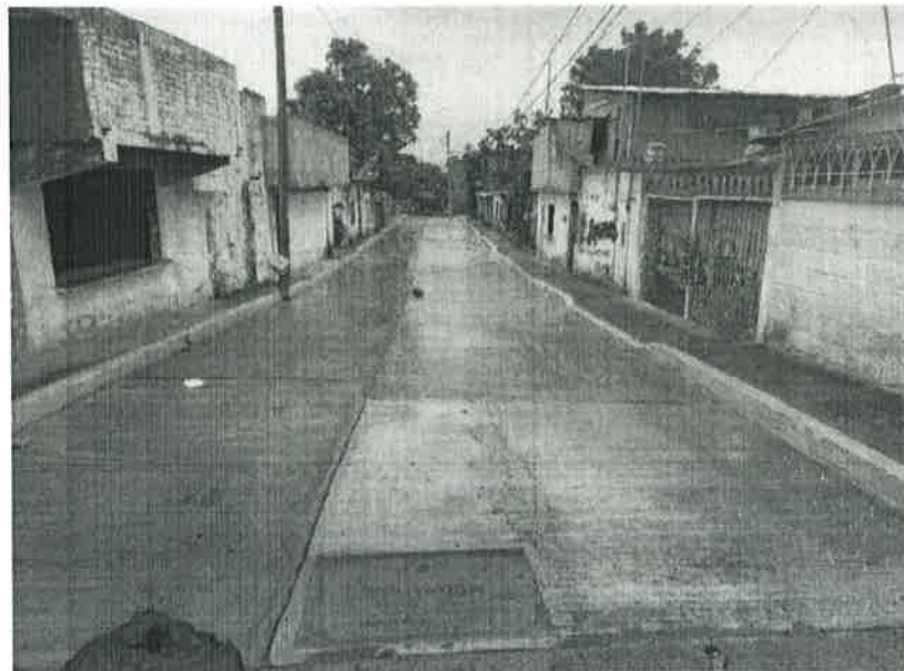
Concepto de obra ejecutado: Construcción de pavimento hidráulico de 18 CM de espesor
