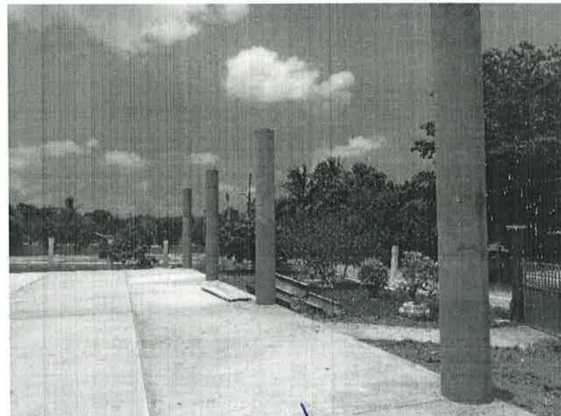
Concepto de obra ejecutado: Construcción de columnas de concreto armado f_c = 200 \text{ Kg/cm}^2 de 45 CM de diámetro.
