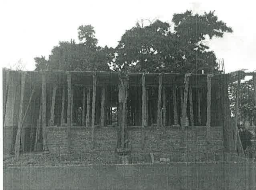
Concepto de obra ejecutado: En la fotografía se aprecia el habilitado de cimbra para construcción de losa de concreto armado.
