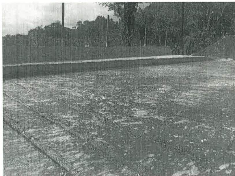
Concepto de obra ejecutado: La fotografía muestra la construcción de pavimento de concreto hidráulico en el punto indicado.
