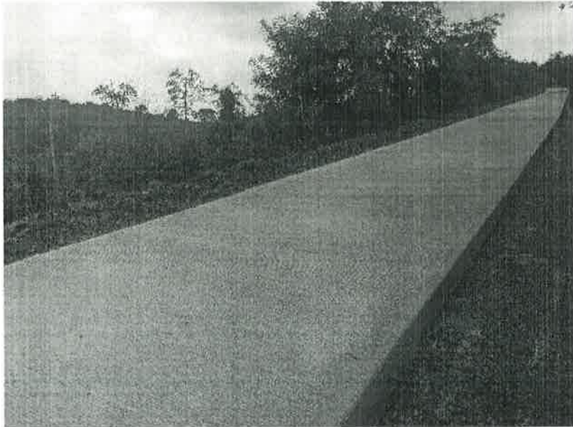
Concepto de obra ejecutado: Pavimento de concreto hidraulico fc=250kg//cm2
