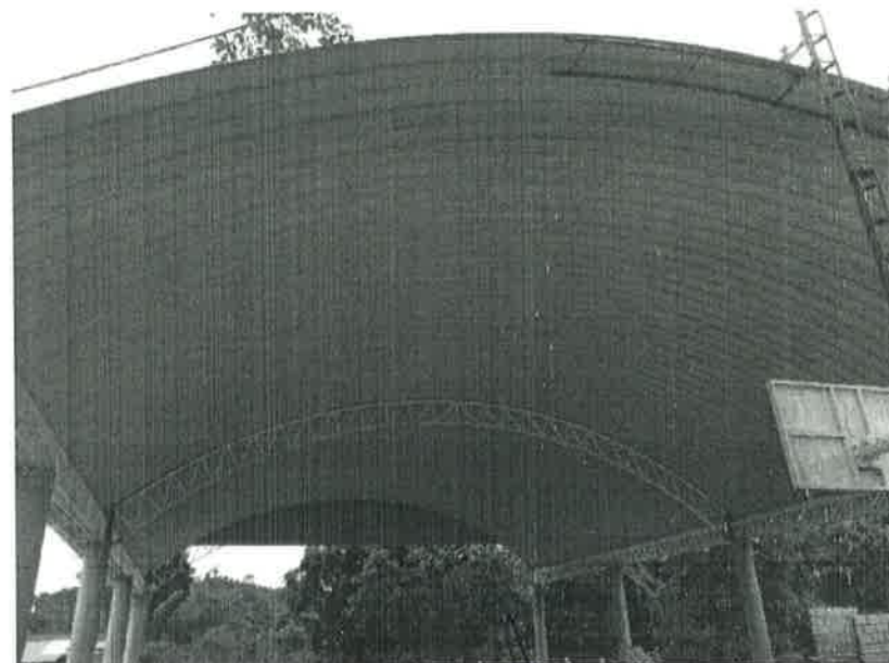
Concepto de obra ejecutado: Suministro y colocacion de lámina rolada en sitio cal. 22 autosoportante
